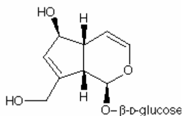
Fig 25. Aucubin
