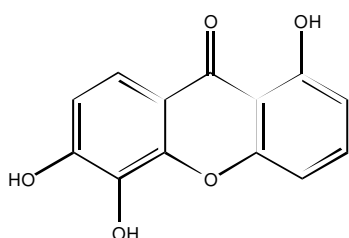
Fig 29. Mesuazanthone-B
