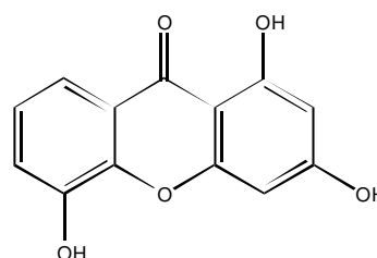
Fig 30. Mesuazanthone-A
