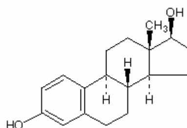
Fig.15 Estradiol
